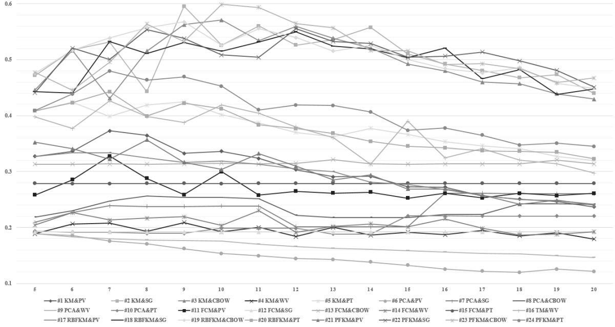
Figure. 4. F1 validation results.
