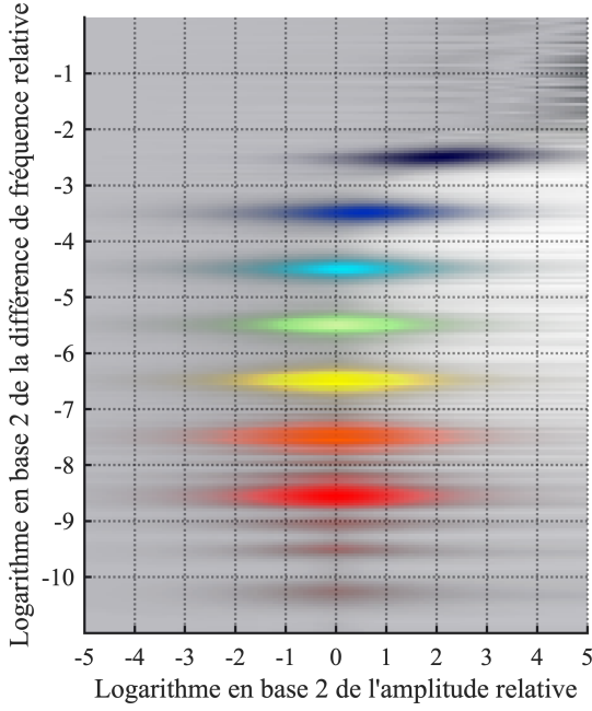
FIGURE 1 – Carte de chaleur du coefficient de masquage lors de la diffusion en ondelettes de deux composantes sinusoïdales x_1 et x_2 , mesuré autour de la fréquence f_1 , et évoluant en fonction de l’amplitude relative \frac{a_2}{a_1} et de la différence de fréquence relative \frac{|f_2 - f_1|}{f_1} . La couleur de chaque tache de diffusion indique la la résolution d’analyse \lambda_2 de la deuxième strate du réseau. Les ondelettes de diffusion ont un profil asymétrique (gammatone) et un facteur de qualité Q = 4 . Elles couvrent un intervalle total de neuf octaves en-deçà de f_1 . Par souci de clarté, on affiche une seule interférence par octave au lieu de quatre.
