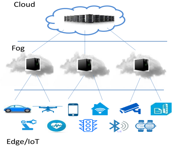
Fig. 2: Fog Overview
