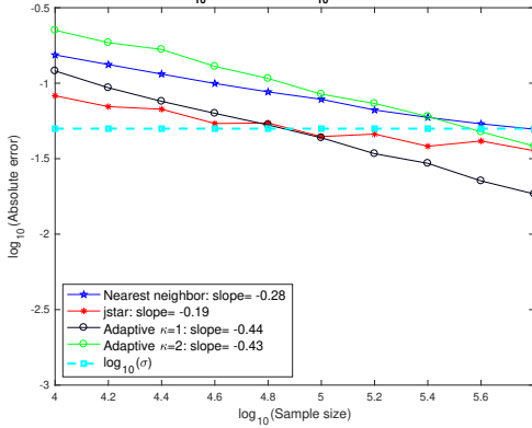
(d) the 3-dim Z-manifold, \sigma = 0.05
