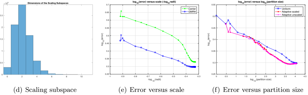
(d) Scaling subspace
