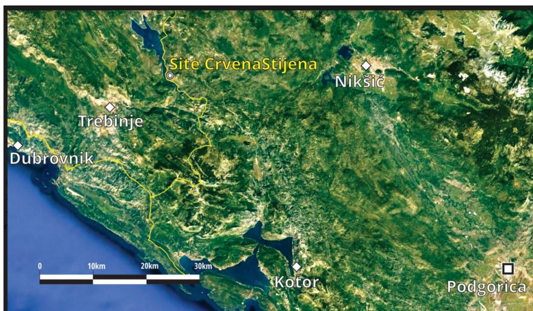
Slika 1A: položaj Crvene Stijene na reljefnoj mapi.
