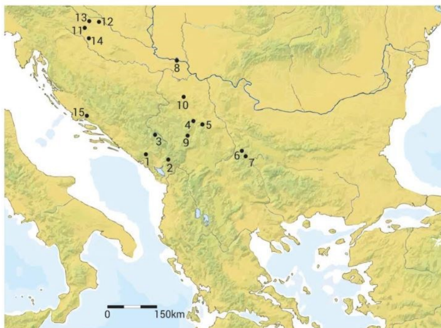
Map of sites: 1. Crvena Stijena, 2. Bioče, 3. Mališina Stijena, 4. Kosovska Kosa, 5. Samaila, 6. Balanica cave, 7. Pešturina cave, 8. Petrovaradin Fortress, 9. Hadži prodanova cave, 10. Šalitrena Pečina, 11. Krapina, 12. Vindija, 13. Velika Pečina, 14. Veternica cave, 15. Mujina Pečina
