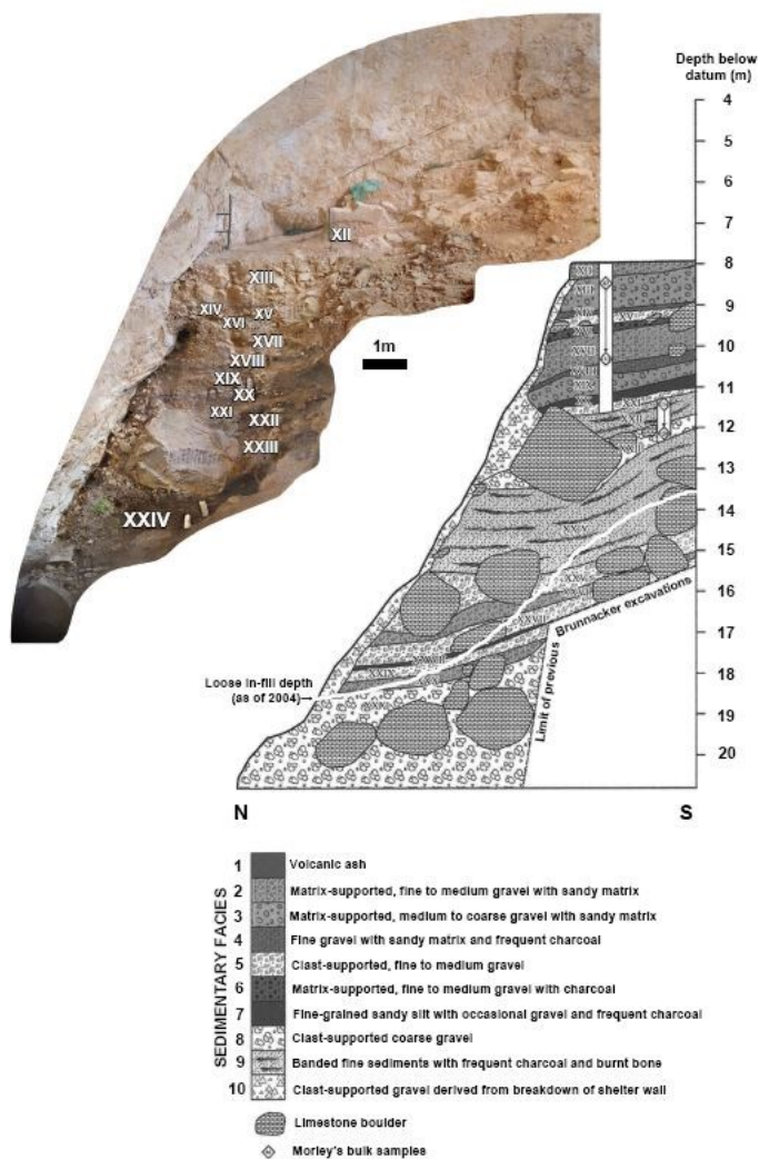
Slika 4: Stratigrafija srednjeg paleolita na Crvenoj Stijeni.
