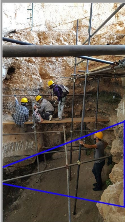
Slika 5: Stratifikovane karakteristike sagorevanja na Crvenoj Stijeni.
