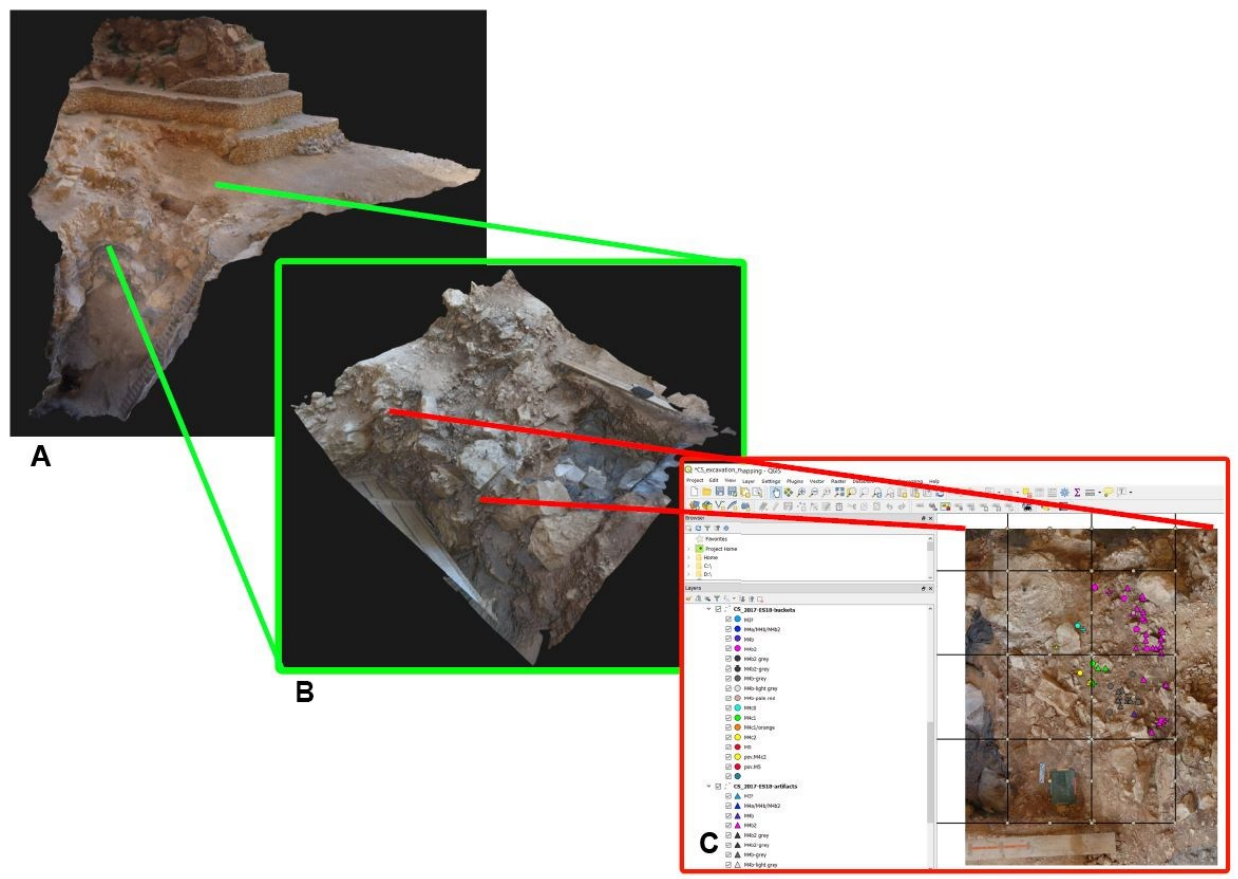
Slika 6. Strategija 3D proveniranja primenjena na Creni Stijena (2017-2019).
