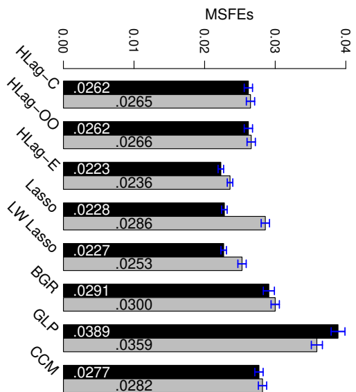
Scenario 3: Elementwise
