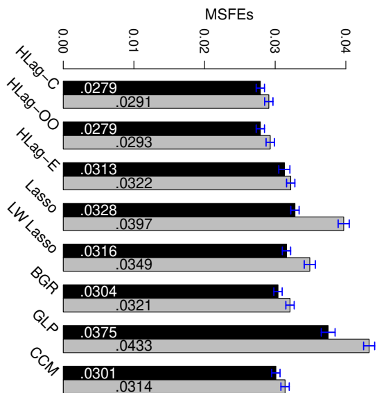
Scenario 1 : Componentwise
