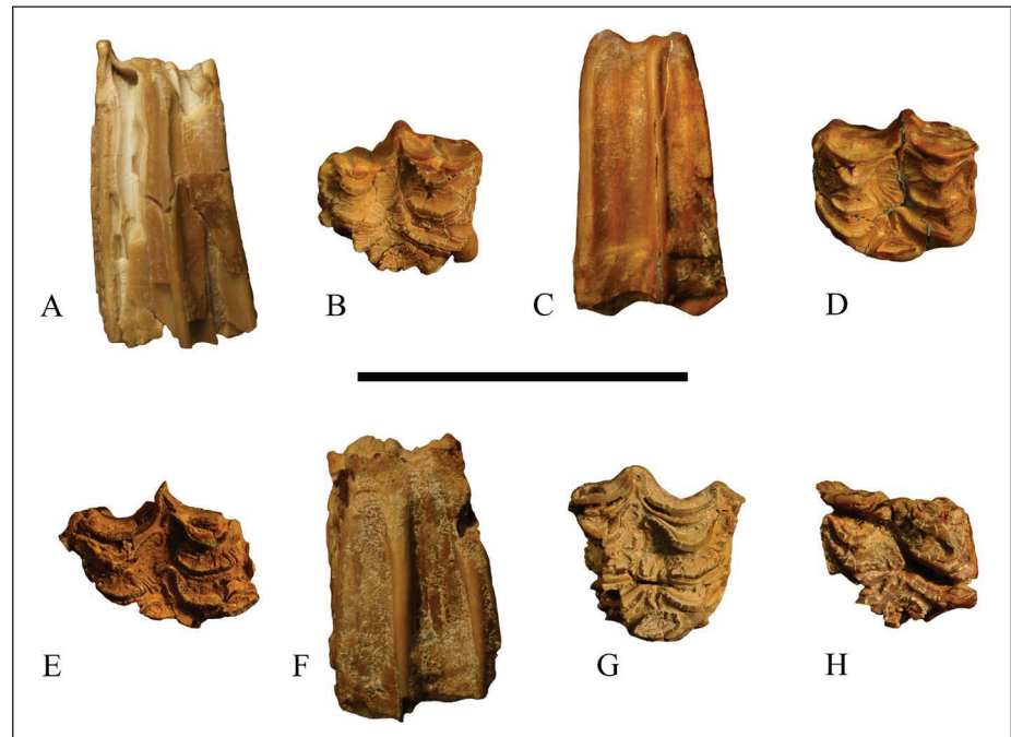
Fig. 11 - Sahabi Eurygnathohippus feibeli P4; ISP85P24A: A) labial, B) occlusal; ISP1P85A: C) labial, D) occlusal; ISP130P16A: E) occlusal; ISP35P99A: F) labial, G) occlusal; ISP78P17A: H) occlusal. Scale bar 5 cm.
