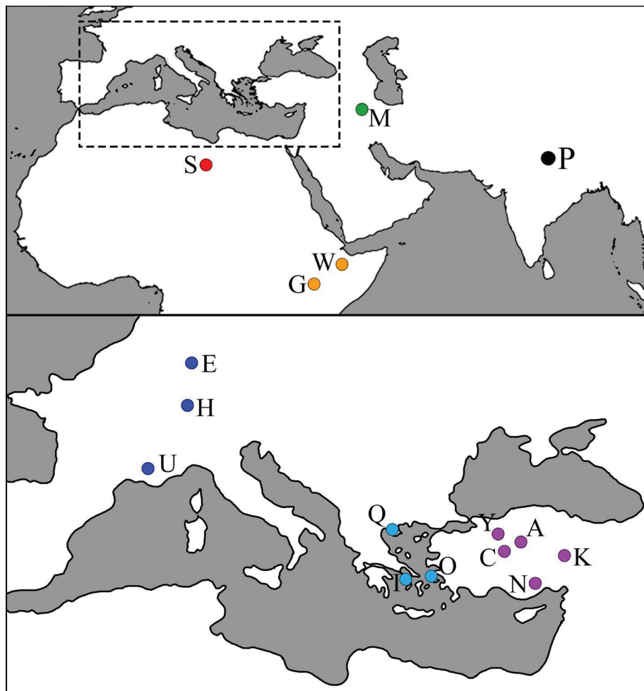
Fig. 1 - Geographical Locator Map: A) Akkasdagi; C) Calta; E) Eppelsheim; G) Lothagam; H) Hoewenegg; I) Pikermi; K) Kurutlu; U) Mt. Luberon; M) Maragheh; N) Sinap & Esme Acakoy; O) Samos; P) Potwar Plateau; Q) Saloniki; S) Sahabi; W) Awash; Y) Corak Yerler.
