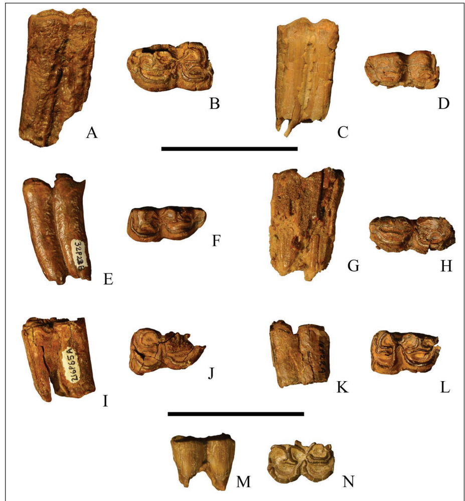
Fig. 15 - Sahabi Eurygnathohippus feibeli m1, ISP3P34B: A) labial, B) occlusal; ISP86P24: C) labial, D) occlusal; ISP32P28: E) labial, F) occlusal; ISP-71P103A: G) labial, H) occlusal; ISP216P65A: I) labial, J) occlusal; ISP16P22A: K) labial, L) occlusal; ISP-195P16A: M) labial, N) occlusal. Scale bar 5 cm.
