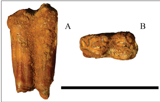
Fig. 16 - Sahabi Eurygnathohippus feibeli m2, ISP81P103A: A) labial, B) occlusal. Scale bar 5 cm.
