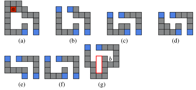
Fig. 2 (a) Start gadget (b) Assignment gadget (c) Positive gadget (d) Negative gadget (e) Buffer gadget (f) Notch gadget (g) Goal gadget
