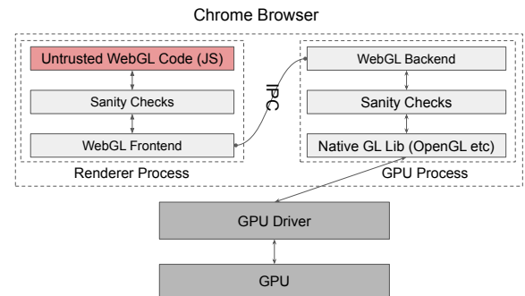
Figure 1: Chrome’s WebGL implementation.
