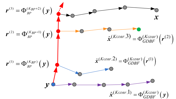
Sl 2. Ilustracija prve strategije, osnova je GDBF w/m algoritam, dok procena nakon odgovarajuće iteracije SPA algoritma određuje referencu.
