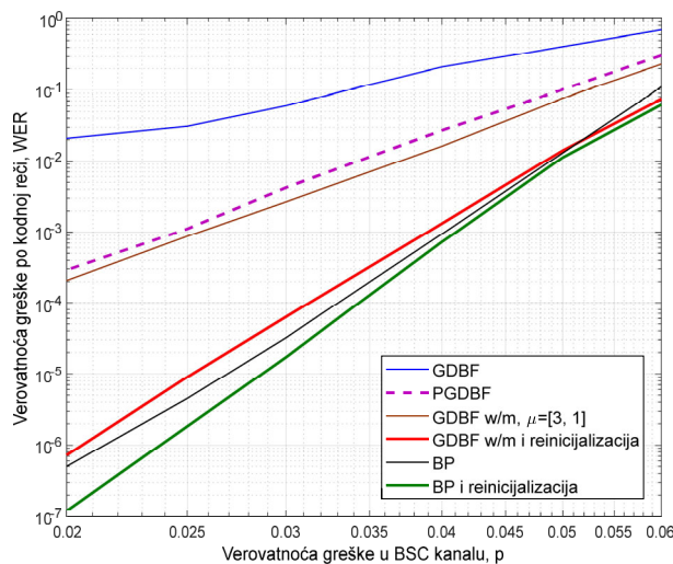
Sl. 6. Zavisnost verovatnoće greške po kodnoj reči od verovatnoće greške u BSC, za Tanerov kod (115,64) i L=300 . Prikazane su performanse za GDBF-w/m i BP, kao i dve strategije njihovog kombinovanja.
