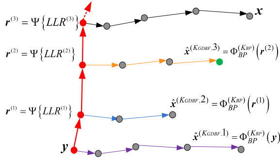
Sl. 3. Ilustracija prve strategije, osnova je GDBF w/m algoritam, dok procena nakon odgovarajuće iteracije SPA algoritma određuje referencu.
