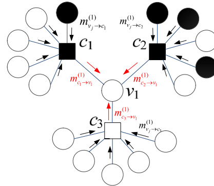
SI 1. Ilustracija BP algoritma na grafu koji odgovara regularnom kodu sa parametrima \gamma=3, \rho=5 .
