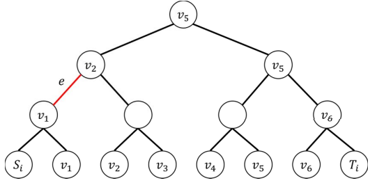
(a) The red edge e contains an edge in F .
