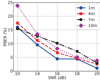
(d) VarAmp at Lab
