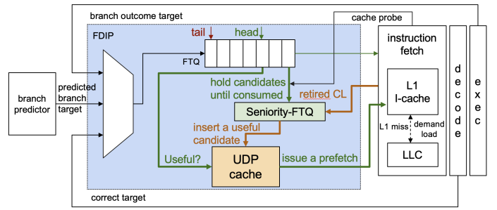
Fig. 10. UDP Microarchitecture
