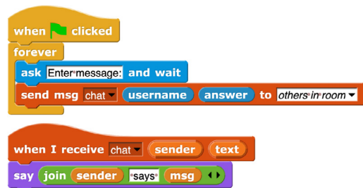
Fig. 9. Simple chat app.
