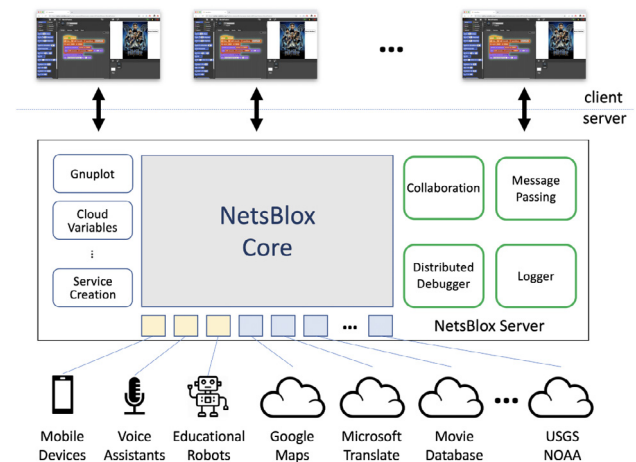
Fig. 27. NetsBlox architecture.
