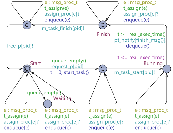
Fig. 5. Front-end model of a PE
