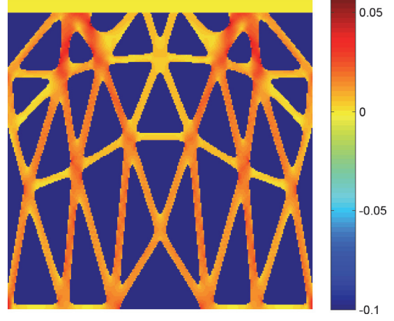
(d) The stress distribution
