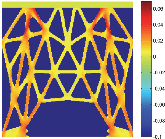
(d) The stress distribution
