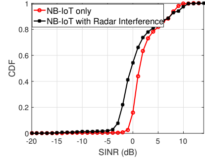
Fig. 5: CDF of SINR.
