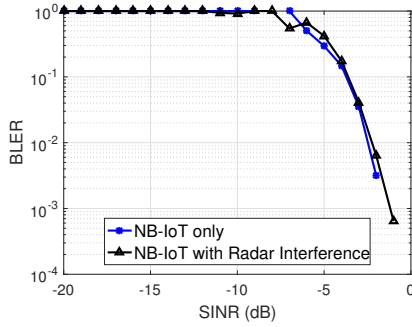
Fig. 4: BLER versus SINR (Uplink).
