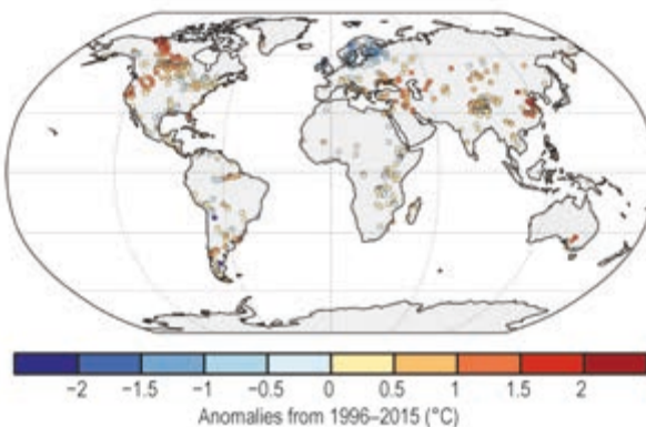
(d) Warm Nights (TN90p)
