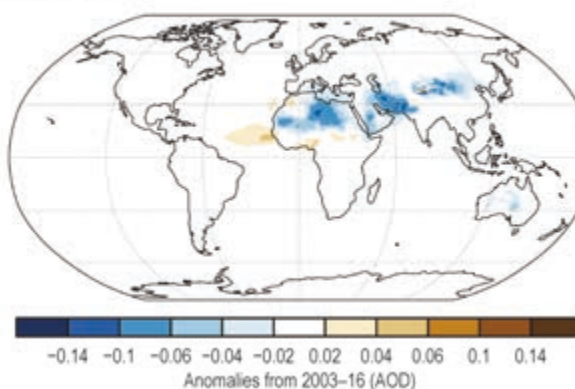
(aa) Dust Aerosol
