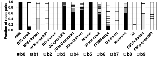
Fig. 10. Inter-wavefront data reuse.
