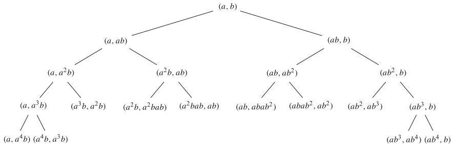
Fig. 3 The tree of Christoffel pairs
