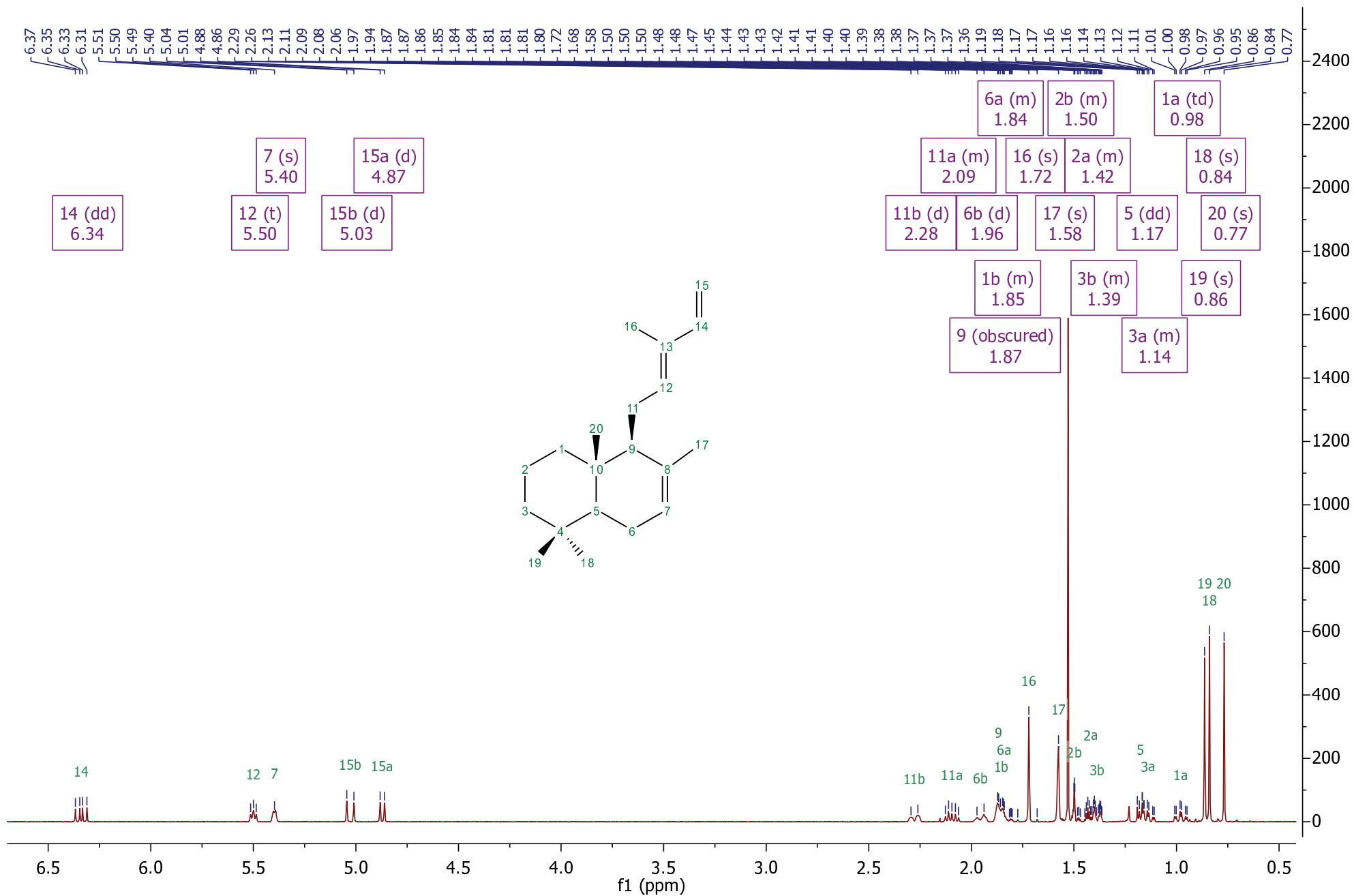
Figure S13-A. ^1\text{H} NMR of labda-7,12E,14-triene [24].
