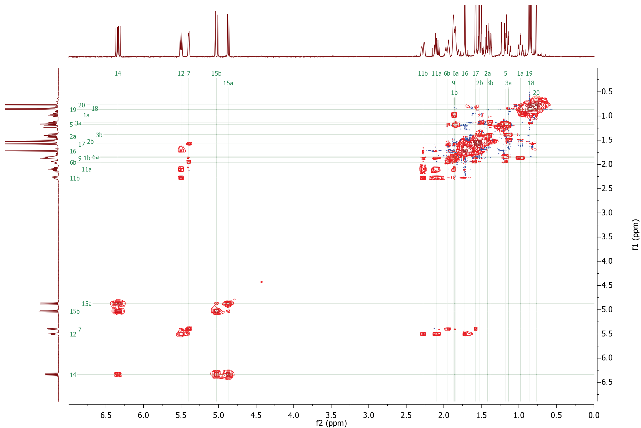
Figure S13-C. ^1\text{H} - ^1\text{H} COSY of labda-7,12E,14-triene [24].
