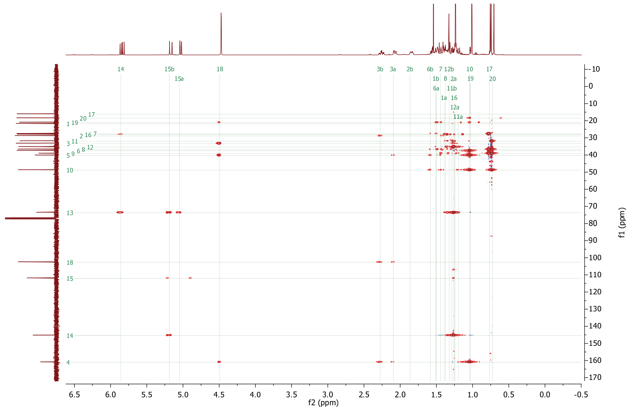
Figure S17-E. ^1\text{H} - ^{13}\text{C} HMBC of neo-cleroda-4(18),14-dien-13-ol [37].
