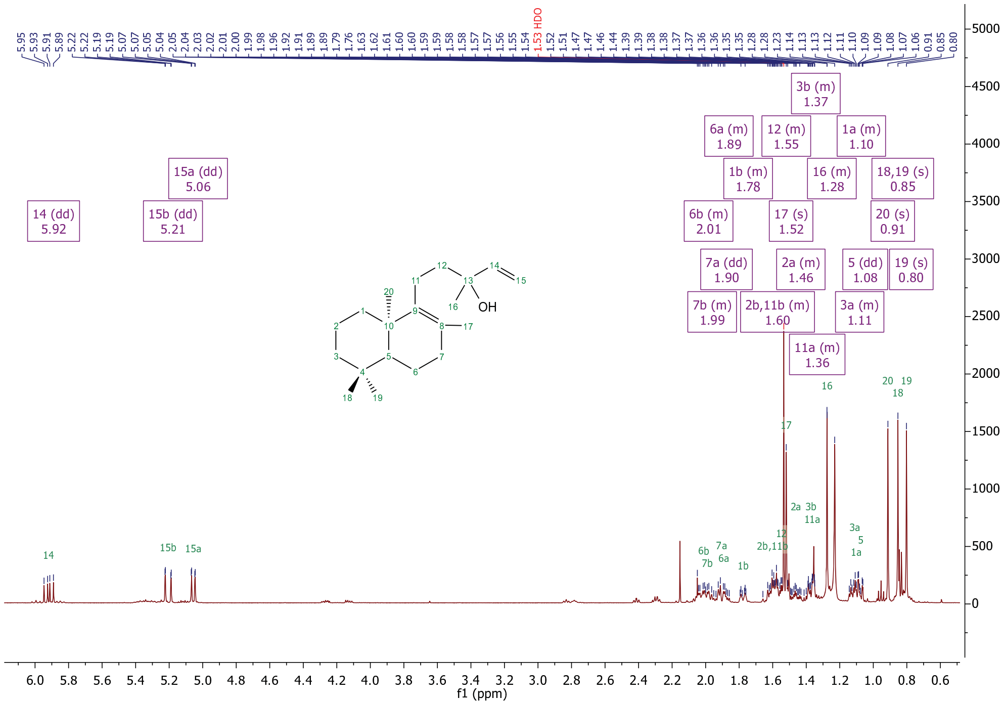
Figure S15-A. ^1\text{H} NMR of (10R)-labda-8,14-dien-13-ol [26].
