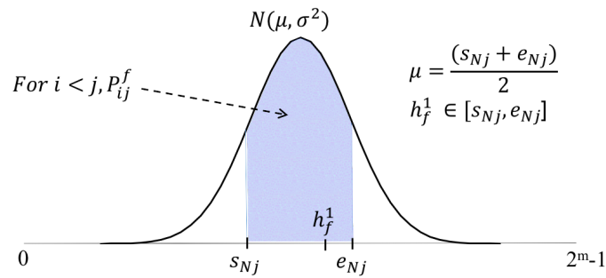
Fig. 6. The function P_{ij}^f
