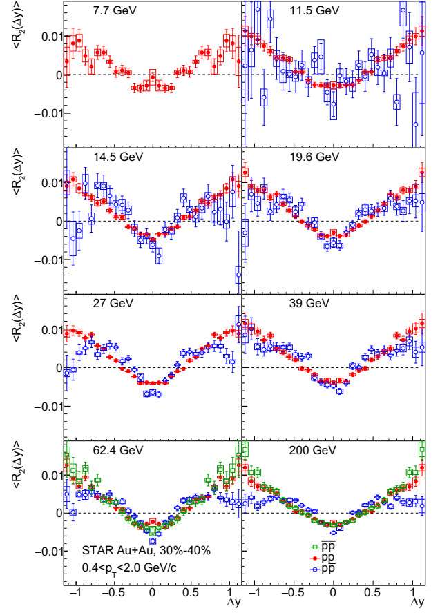
(b) protons
