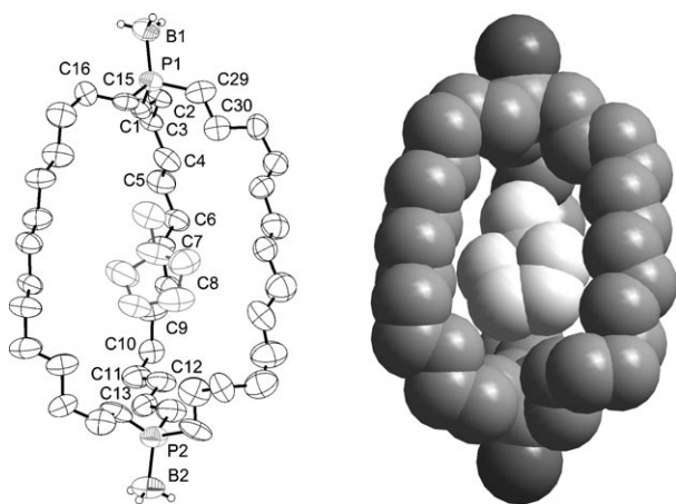
Abbildung 3. Molekülstruktur von out,out -2-2-BH 3 ·(C 5 H 9 CH 3 ). Die Kohlenstoffatome C1–C14 und C15–C18 weisen Fehlordenungen auf, die modelliert werden konnten. Gezeigt ist diejenige Konformation mit den Kohlenstoffatomen der höchsten Aufenthaltswahrscheinlichkeit.
