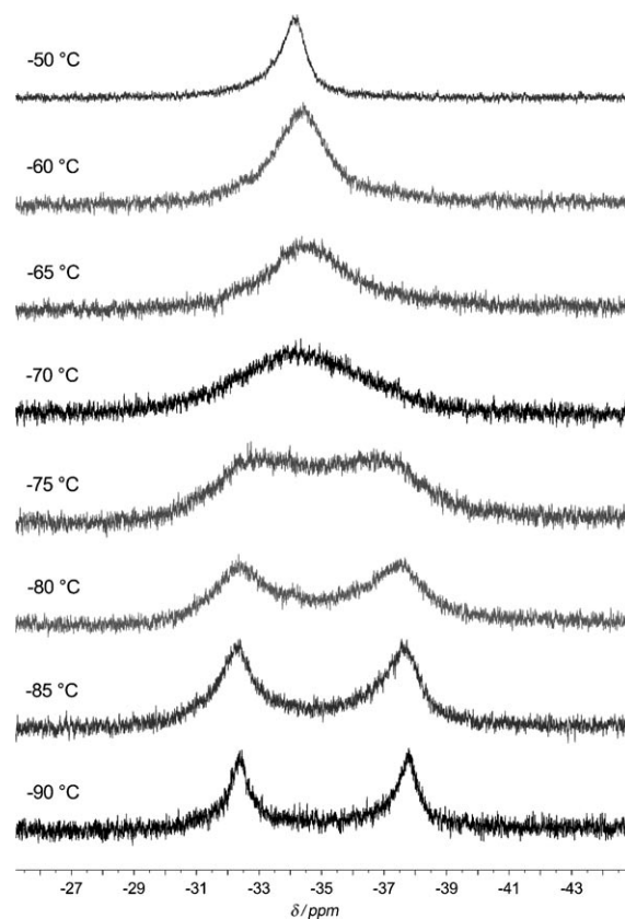
Abbildung 2. ^{31}\text{P}\{^1\text{H}\} -NMR-Spektren von in,out-2 bei niedrigen Temperaturen.
