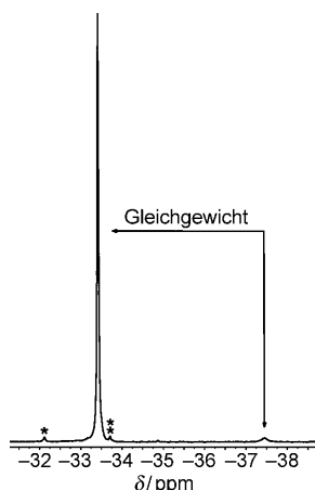
Abbildung 1. ^{31}\text{P}\{^1\text{H}\} -NMR-Spektrum von 2 in [\text{D}_8] -Toluol bei -80^\circ\text{C} (die Pfeile kennzeichnen die beiden miteinander austauschenden Spezies; * und ** zeigen bisher nicht bekannte Nebenprodukte an).
