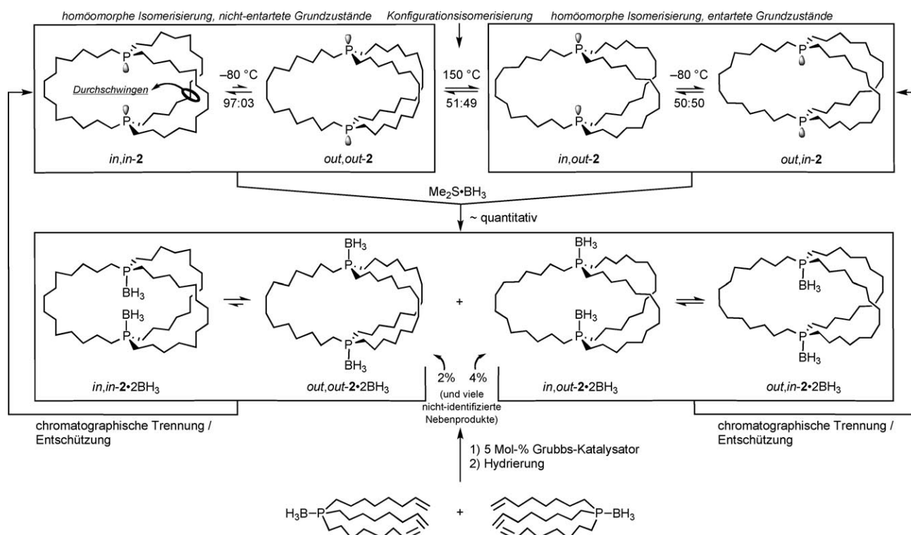
Schema 2. Isomerisierung von 2 und die Synthese der \text{BH}_3 -Addukte.
