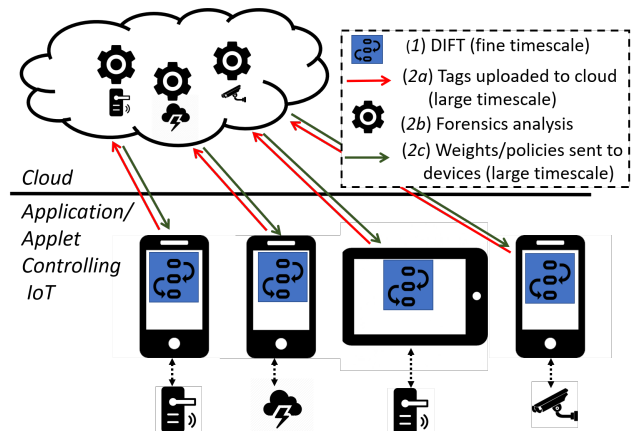
Fig. 1. DDIFT Architecture.
