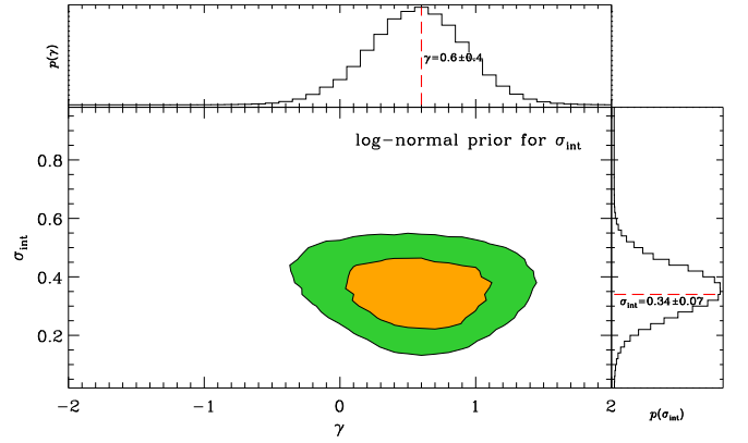
(d) \mathcal{M}_{\text{BH}}\text{-}L_{\text{host}} , lognormal prior
