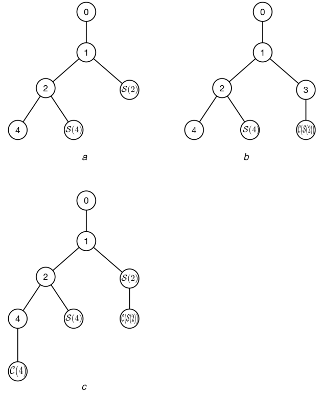
Fig. 21 Proof of Lemma 1
