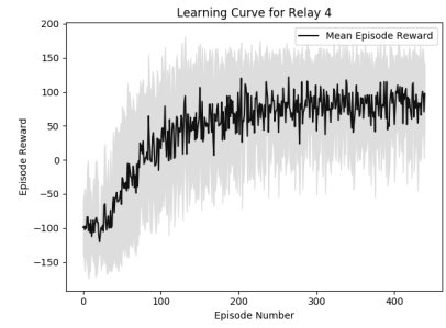
(c) Relay 4: Episodic reward
