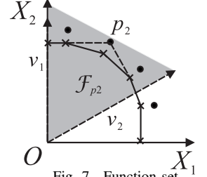
Fig. 7. Function set
