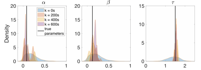
Fig. 3: Posterior parameter PDFs for non-equilibrium driving dataset from PF estimates.
