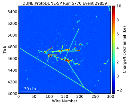
(g) A 6 GeV/ kaon candidate.
