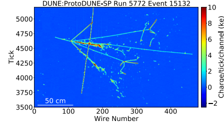
(d) A 6 GeV/ pion candidate.
