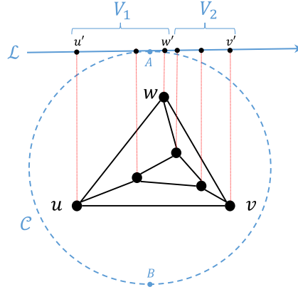
Fig. 2. Proof of Lemma 4.5.
