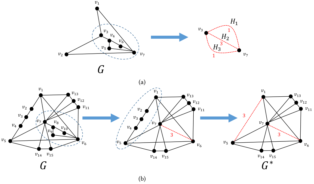
Fig. 5. Lemma 4.15.
