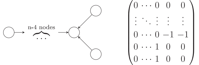
Q2: ['D', n ]
