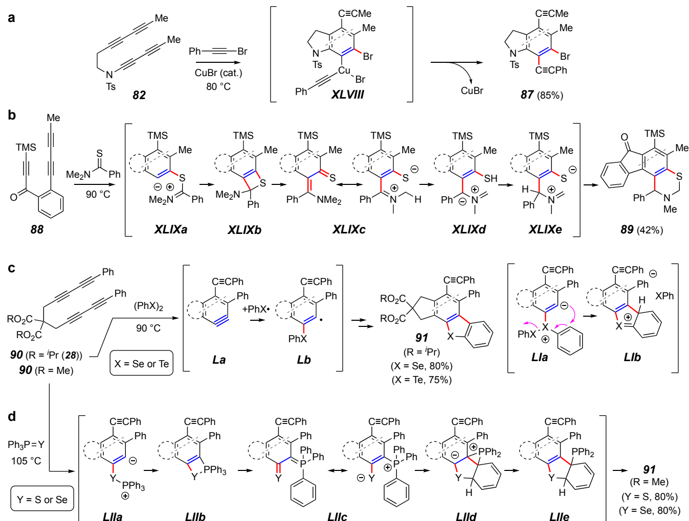
Figure 10. Trapping reactions forming a C–C and a C–Br, C–S, C–Se, or C–Te bond.
