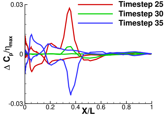
(b) Mode 2
