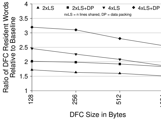
Fig. 12. DFC Data Utilization
