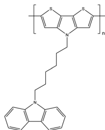
Fig. 1 Poly(4-(6-(9 H -carbazol-9-yl)hexyl)-4 H -dithieno[3,2- b :2',3'- d ]pyrrole) (pC6DTP).
