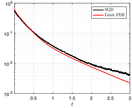
(d) Normalized risk, \delta = 1/10 .
