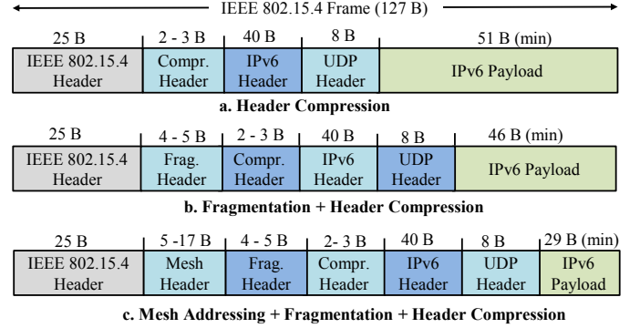
Fig. 6: IEEE 802.15.4 Frame. min = Minimum.
