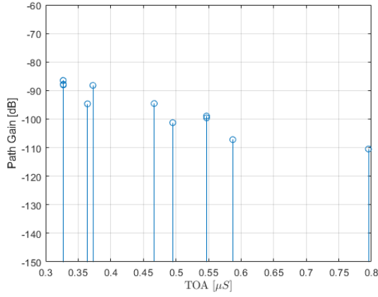
Fig. 3. NLOS scenario CIR.
