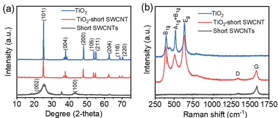
Fig. 2 (a) XRD profiles of TiO 2 , TiO 2 -short SWCNT, and short SWCNTs. (b) Raman spectra of TiO 2 , TiO 2 -short SWCNT, and short SWCNTs.
