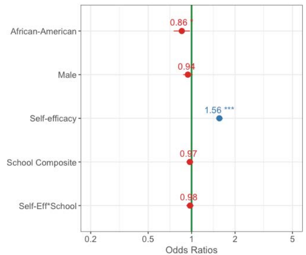
Fig. 3. STEMPATH Model 3
