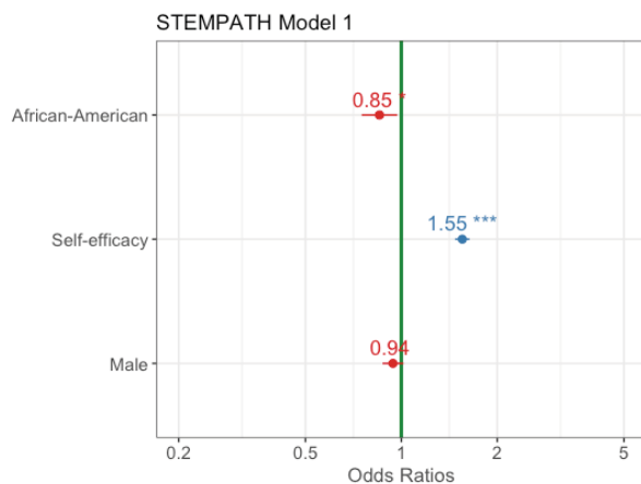
Fig. 1. STEMPATH Model 1
