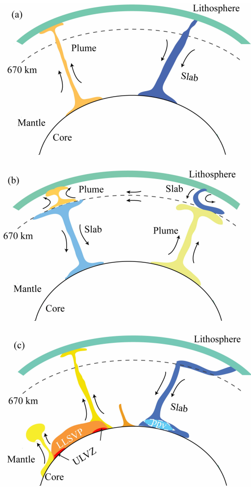
图 5 地幔对流的示意图
