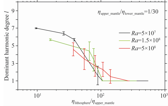
图 11 含有动力边界条件的地幔对流模型得到的地幔结构主导波长和岩石圈平均黏性的关系
