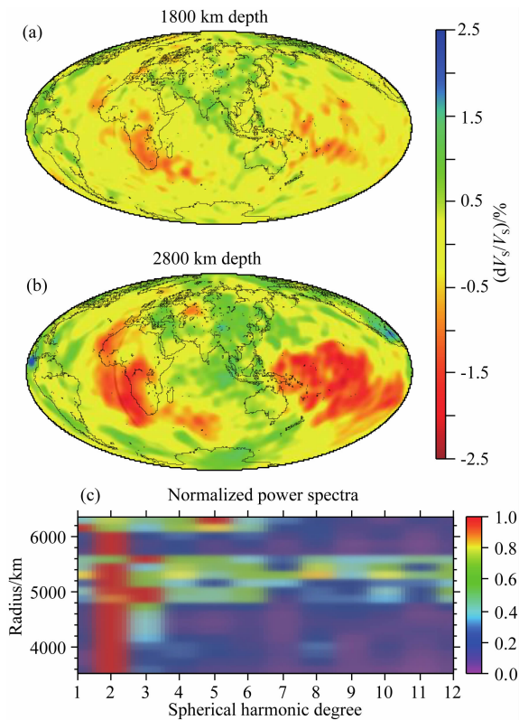
图1 地震层析成像得到的地幔 S 波速度异常 (Ritsema et al. , 2011). 1800 km(a)和 2800 km(b)深度的结构, 及随深度变化的归一化的频谱分布(c). 非洲和太平洋下, 核幔边界上(比如在图 1b, 2800 km 深度上)的低速异常是 LLSVP. 频谱图显示二阶地幔结构的主导性.
