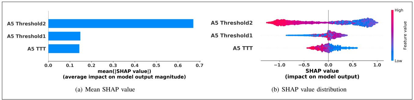
Fig. 6. Impact of each input parameter on RSRP
