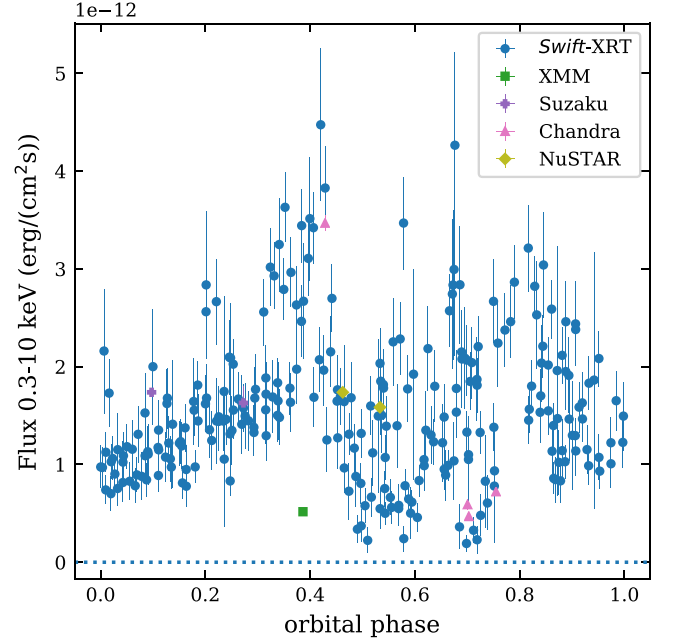
(d) X-rays ( P = 308 days)
