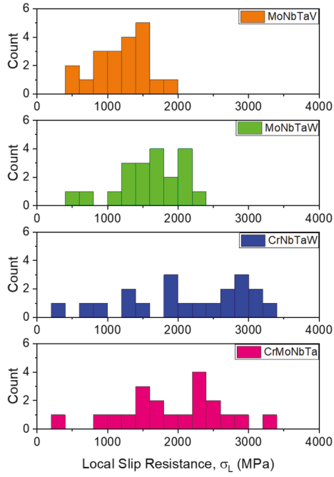
(c) {112} Edge
