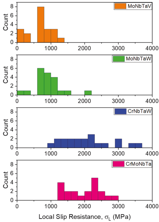
(e) {123} Edge
