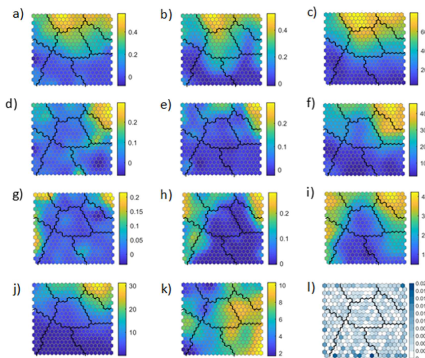
Figure 9: SOM classification: a) \tau_1(Q-P) , b) \tau_2(P-Q) , c) JO(Q-P) , d) \tau_1(Q-SW) , e) \tau_2(SW-Q) , f) JO(Q-SW) , g) \tau_1(P-SW) , h) \tau_2(SW-P) , i) JO(P-SW) , j) JQ(Q-P-SW) , k) SI , l) probability of each SOM centroid.
