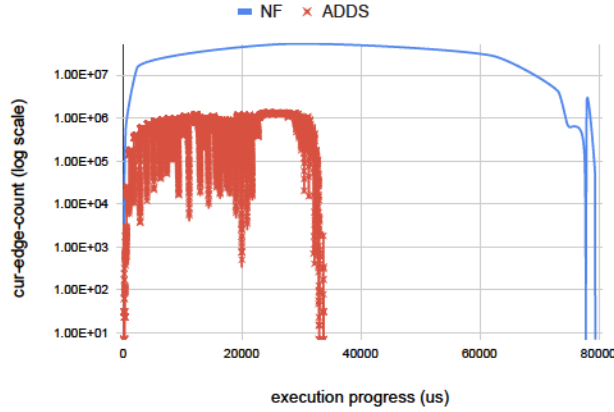
Figure 14. D.mat22: s:2.29×, w:2.18×.
