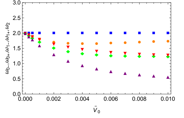
a. N = 10^3 fermions
