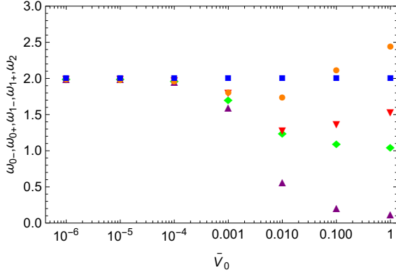
a. N = 10^3 fermions.
