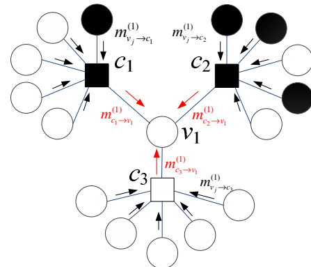
Sl 1. Ilustracija BP algoritma na grafu koji odgovara regularnom kodu sa parametrima \gamma=3 , \rho=5 .
